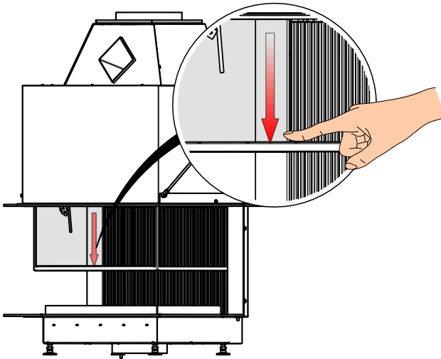
Abb. 1: Funkenschutzgitter
